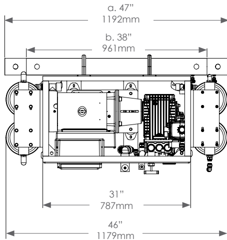
Vessel Assembly a. 2700 / 3200 / 3400 b. 2100 / 2600
