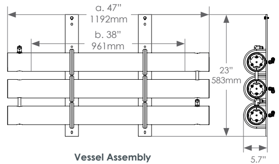
Vessel Assembly a: 2700 / 3200 / 3400 b: 2100 / 2600
